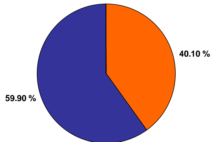
Kapitāls
